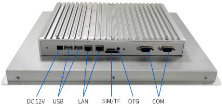
安卓一体机接口及规格
