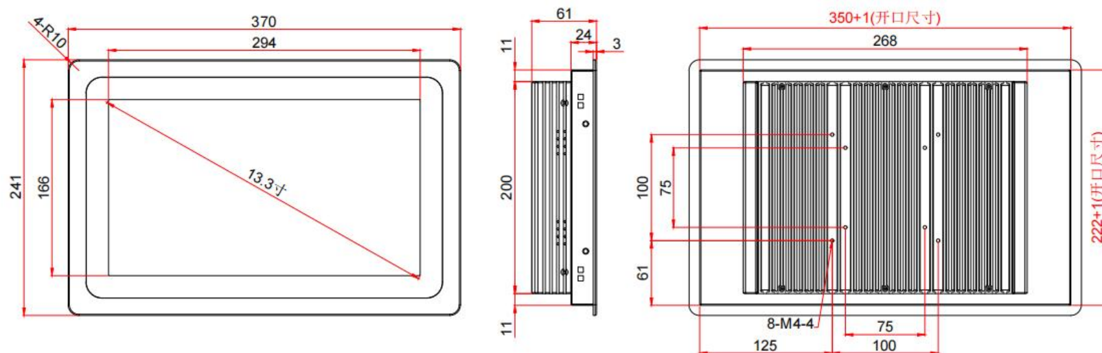
13.3寸外嵌式（全封闭）
