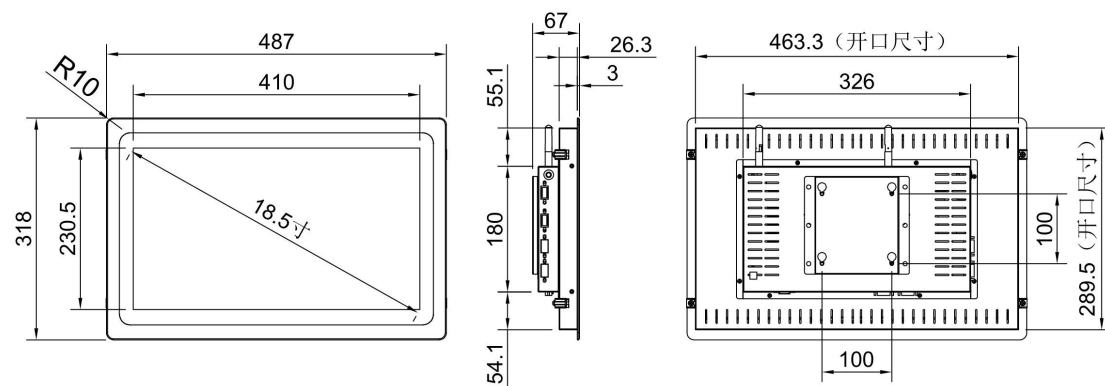
18.5寸外嵌式（散热款）
