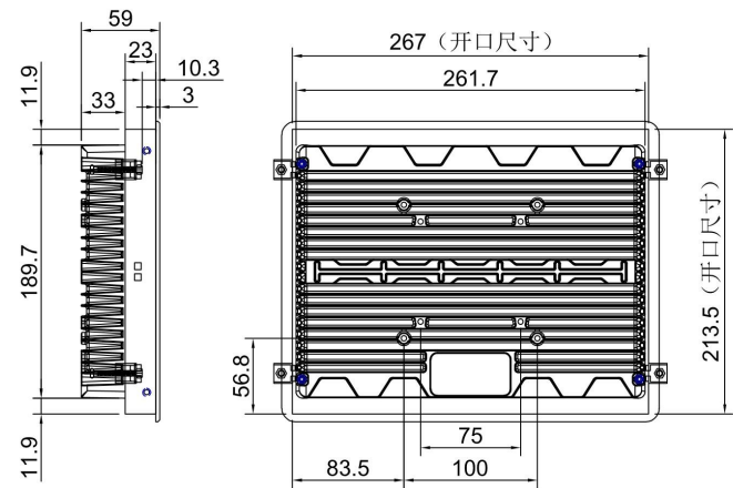
10.4寸外嵌式（全封闭）
