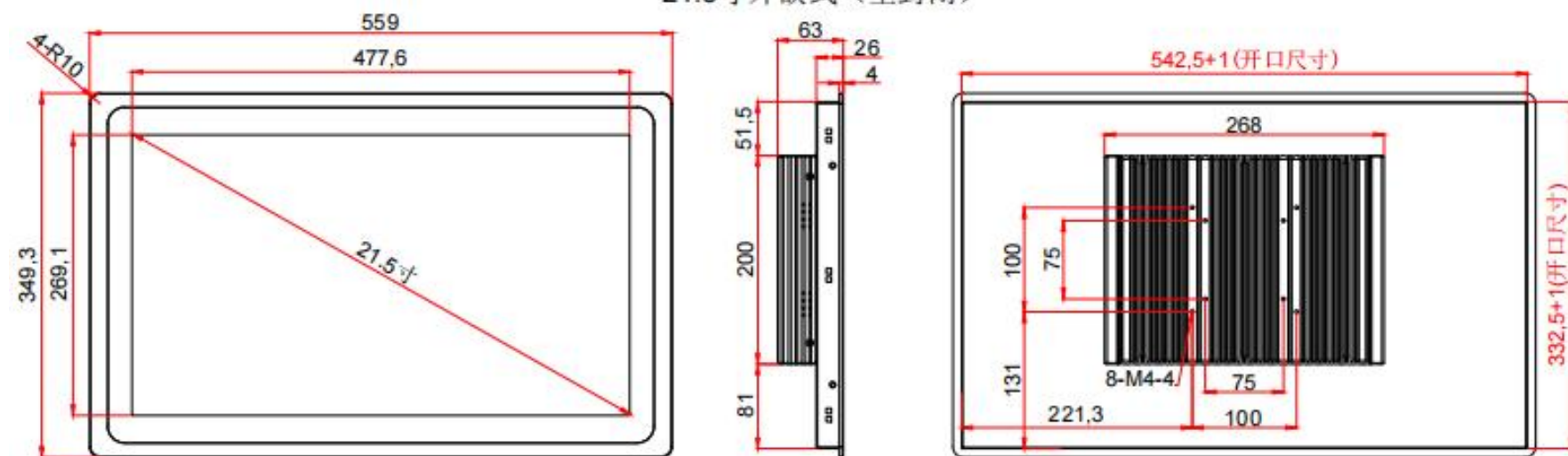
21.5寸外嵌式（全封闭）
