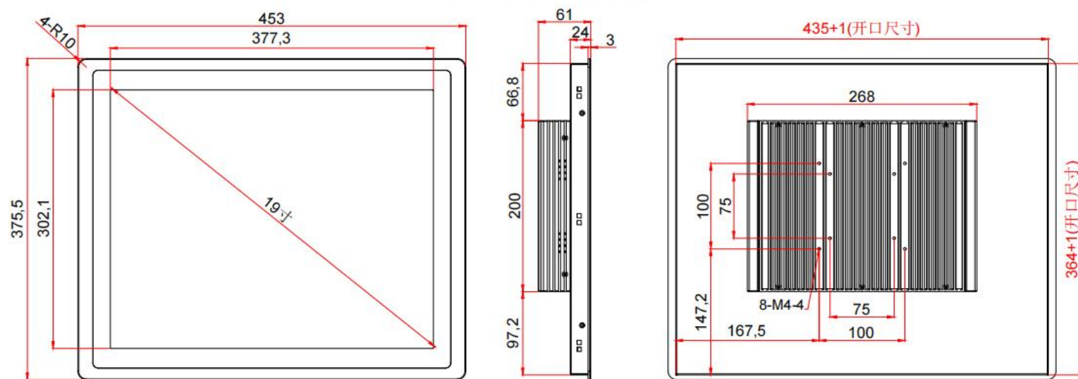
19寸外嵌式（全封闭）
