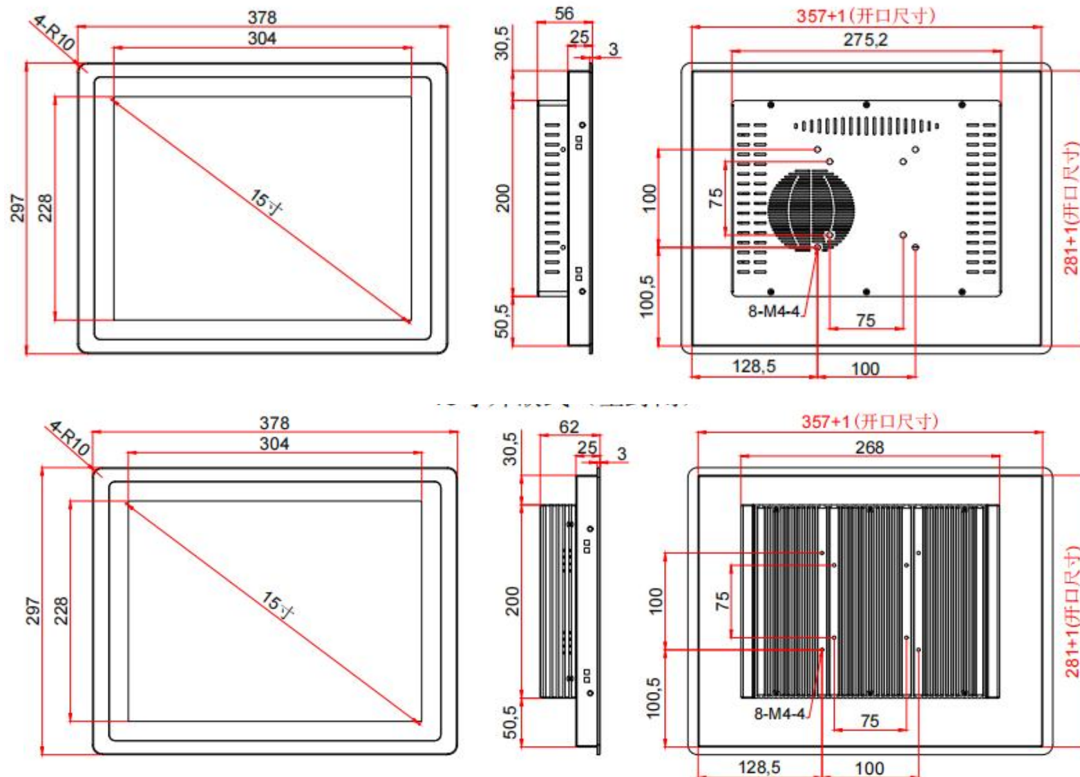
15寸外嵌式（散热款）
