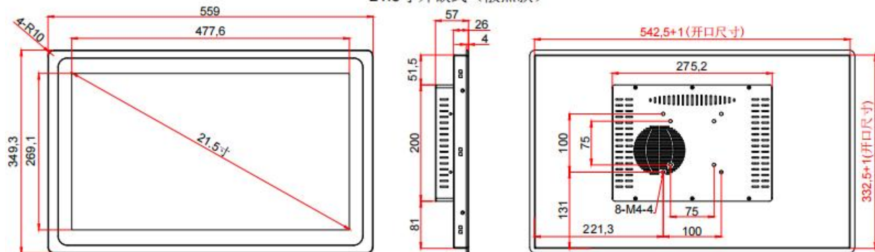
21.5寸外嵌式（散热款）
