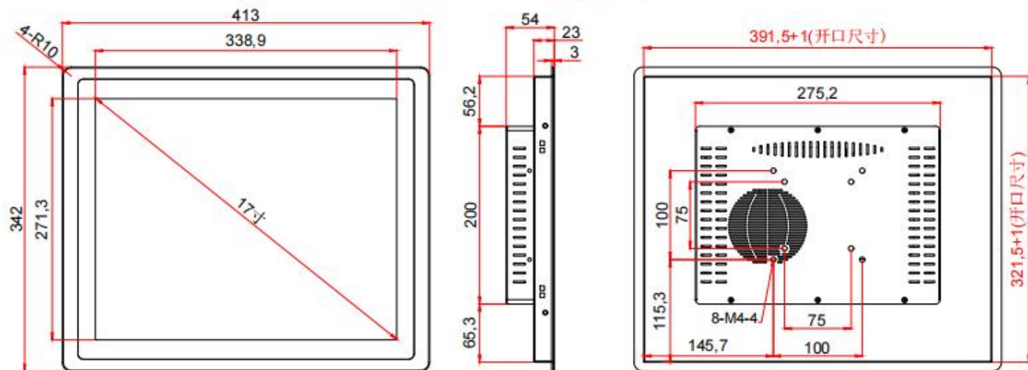
17寸外嵌式（散热款）
