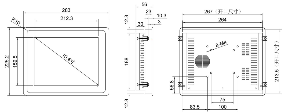
10.4寸外嵌式（散热款）
