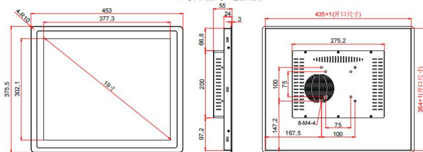
19寸外嵌式（散热款）
