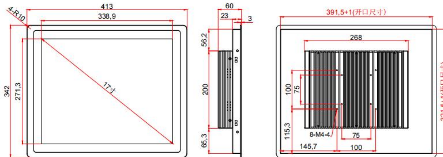
17寸外嵌式（全封闭）
