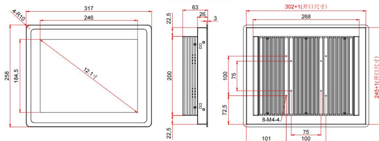
12.1寸外嵌式（全封闭）
