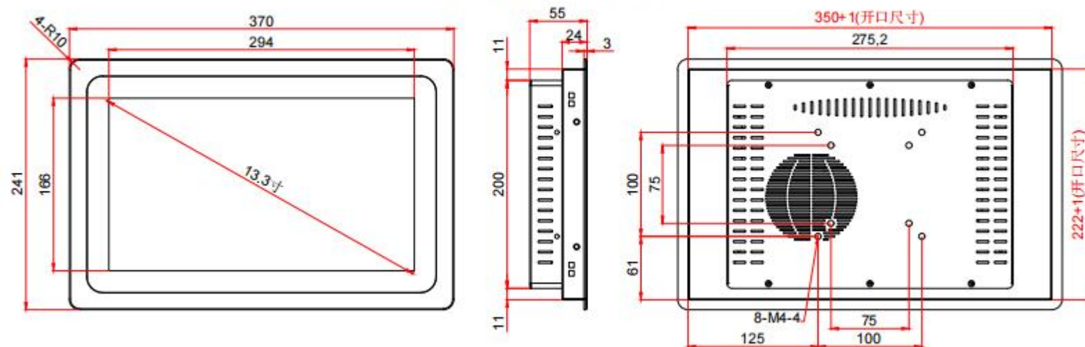
13.3寸外嵌式（散热款）
