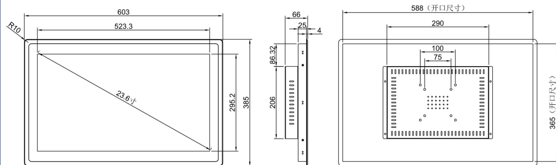
23.6寸外嵌式（散热款）
