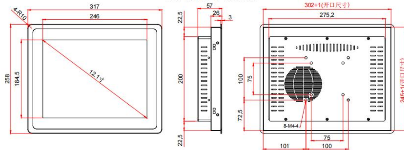
12.1寸外嵌式（散热款）
