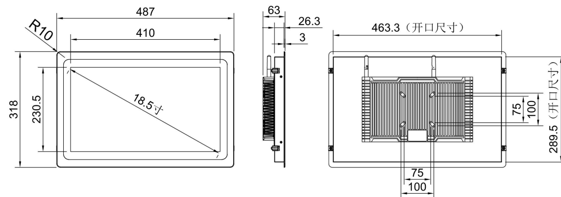
18.5寸外嵌式（全封闭）
