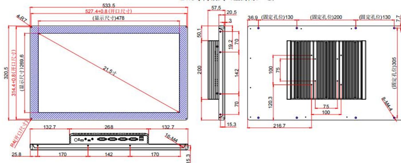
21.5寸内嵌式（散热款）-新
