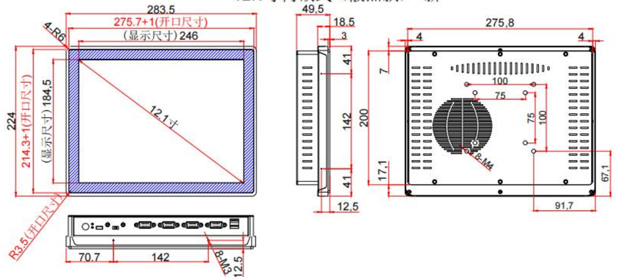
12.1寸内嵌式（散热款）-新
