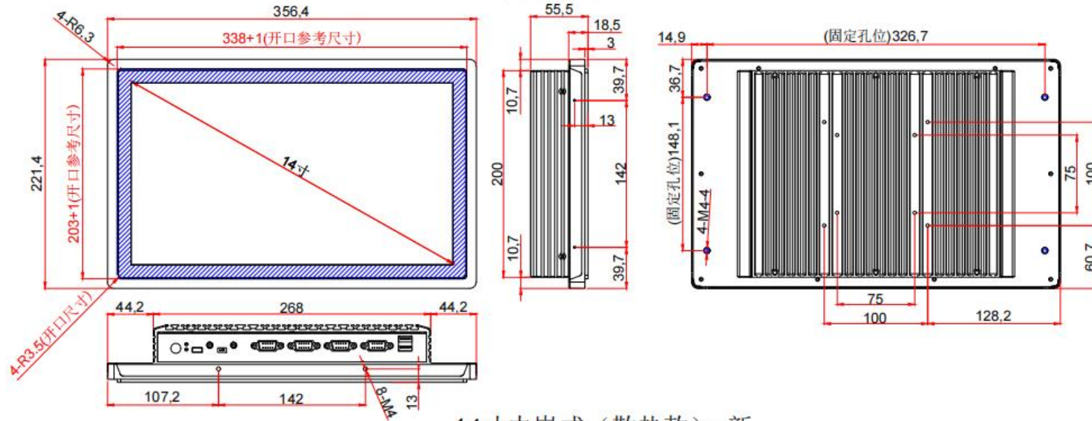
14寸内嵌式（散热款）-新
