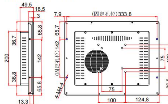
15寸内嵌式（散热款）新
