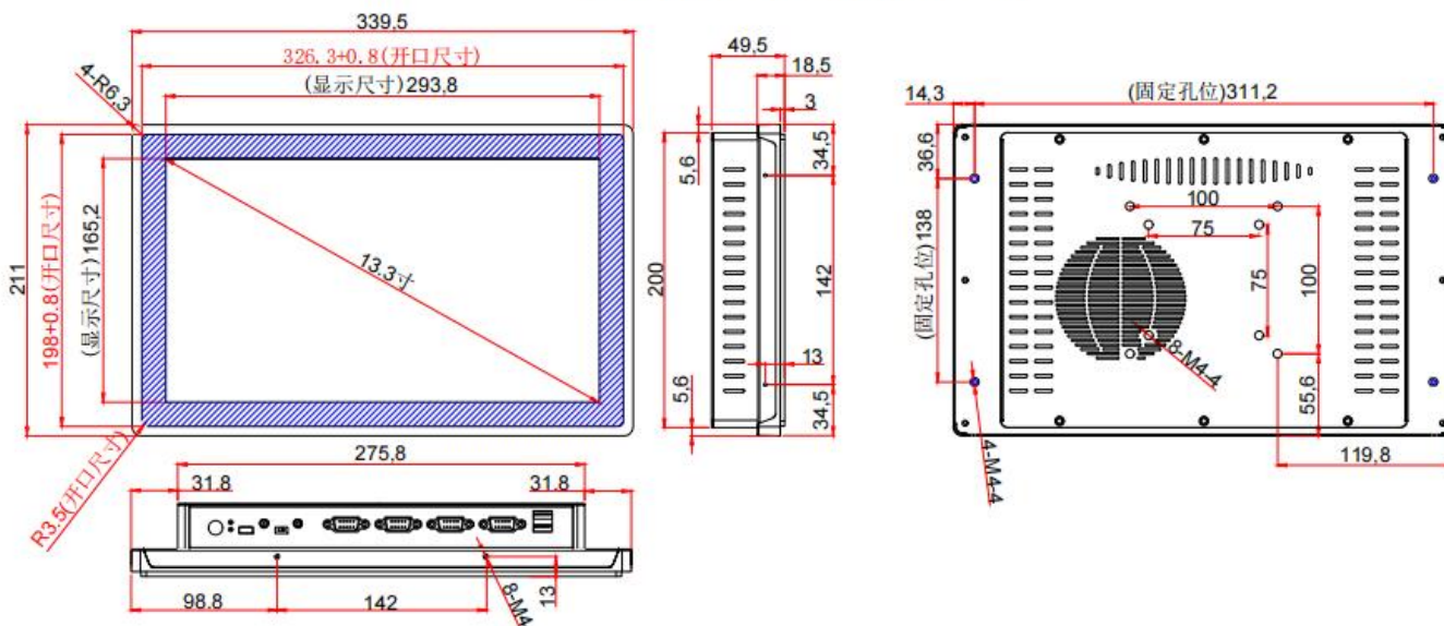
13.3寸内嵌式（散热款）-新
