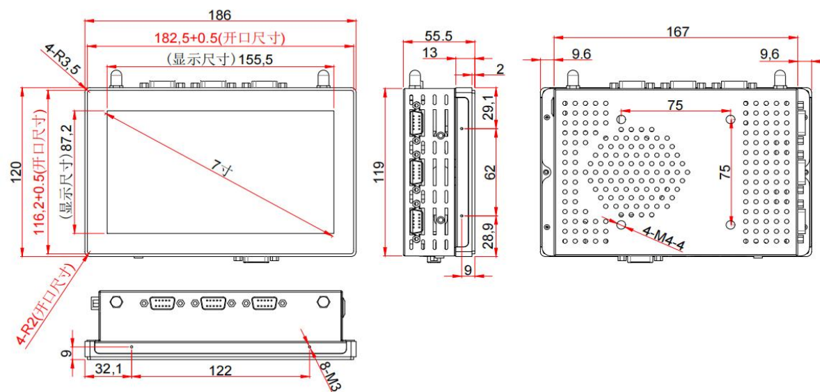
7寸内嵌式（散热款、X86）
