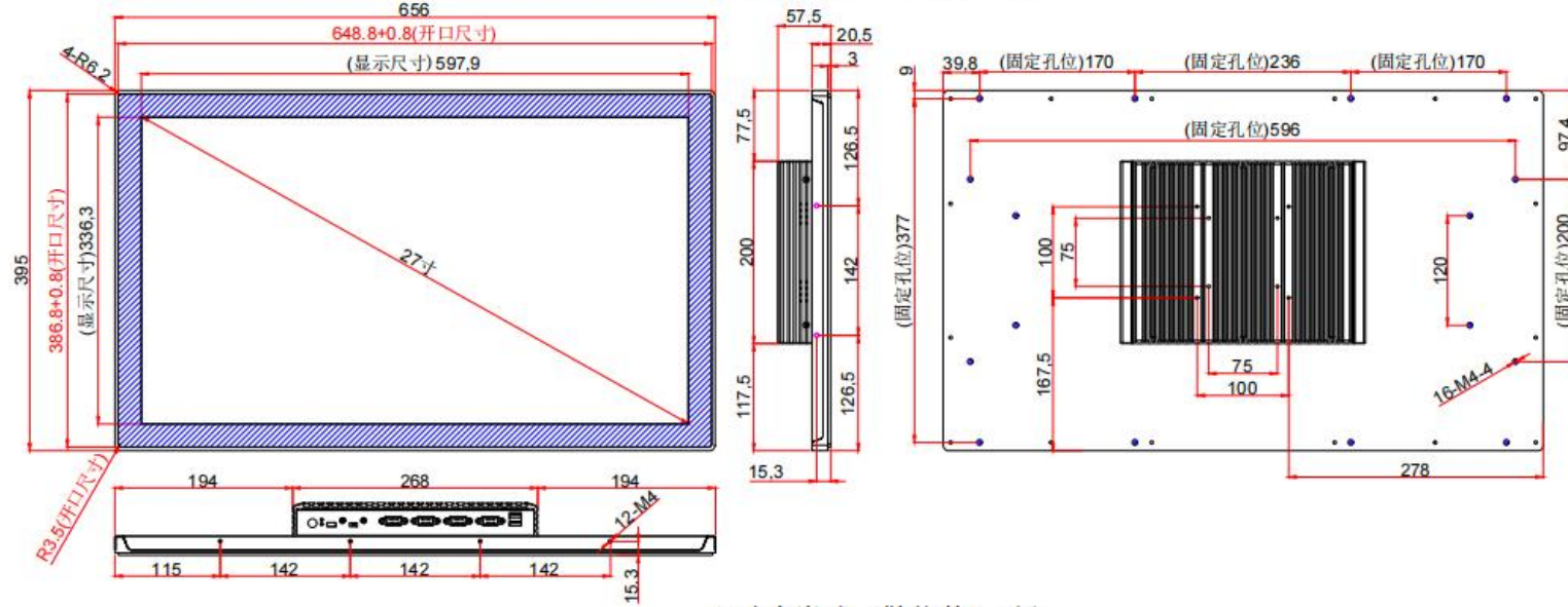
27寸内嵌式（散热款）-新
