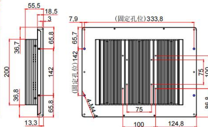
15寸内嵌式（全封闭）-新
