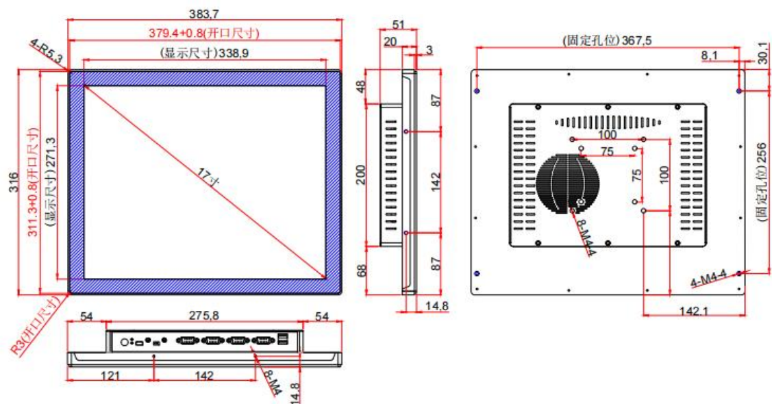
17寸内嵌式（散热款）-新
