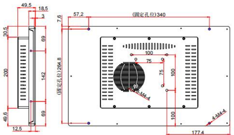
18.5寸内嵌式（散热款）-新
