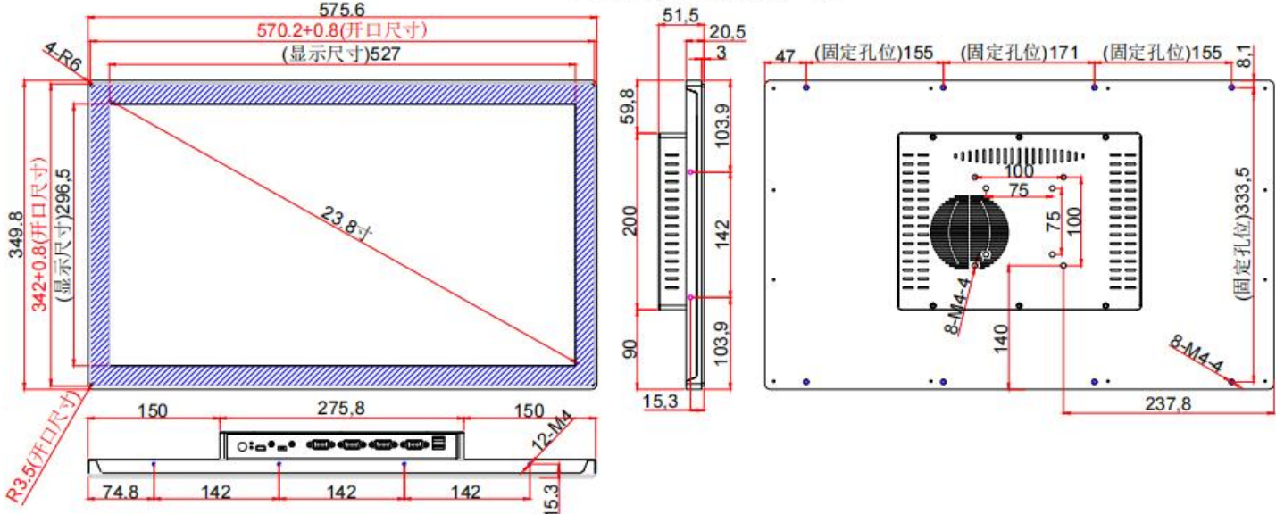
23.8寸内嵌式（散热款）-新
