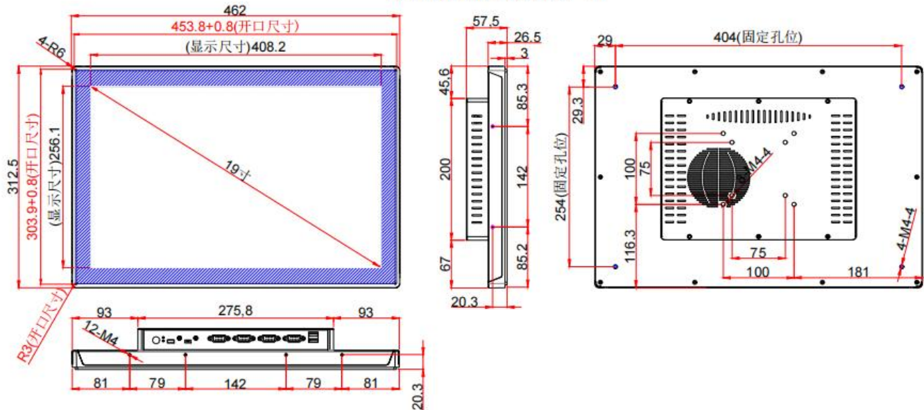
19寸宽屏内嵌式（散热款）-新
