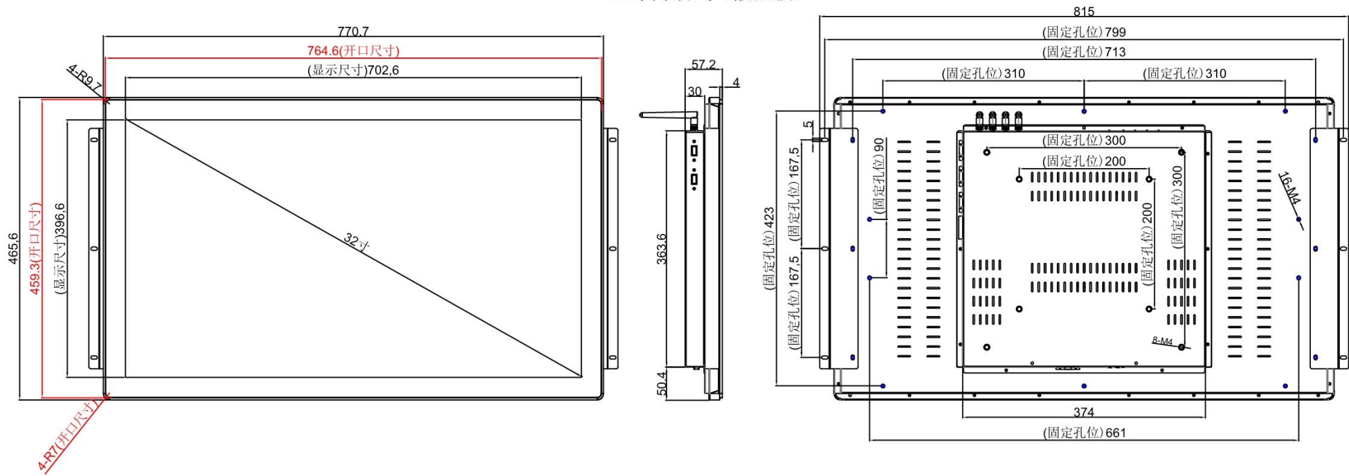
32寸内嵌式（散热款）
