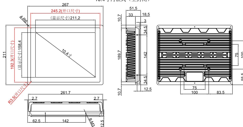
10.4寸内嵌式（全封闭）
