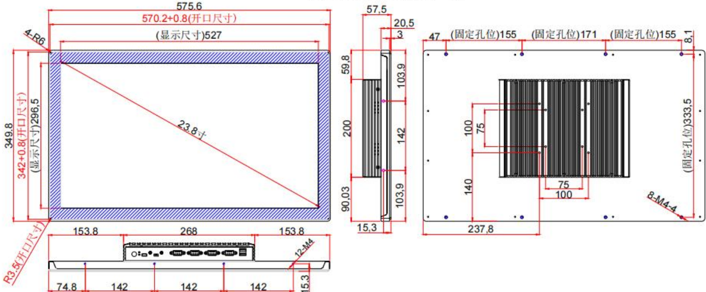
23.8寸内嵌式（散热款）-新
