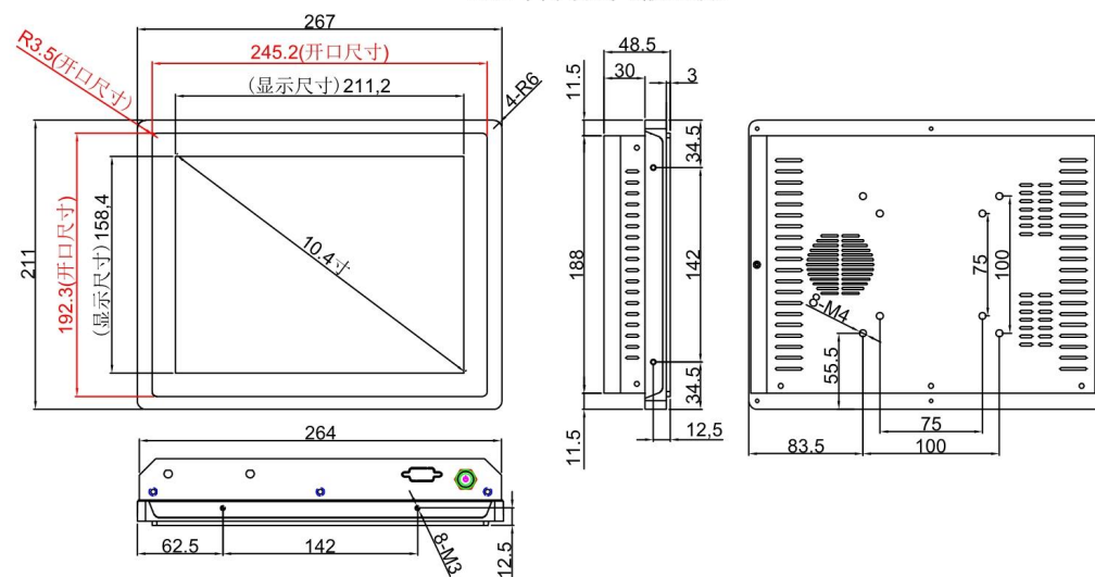
10.4寸内嵌式（散热款）
