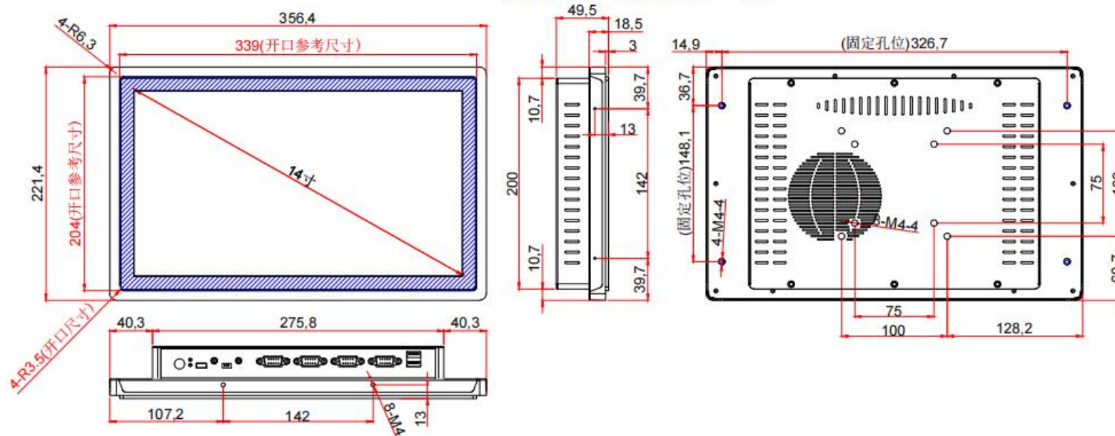
14寸内嵌式（散热款）-新
