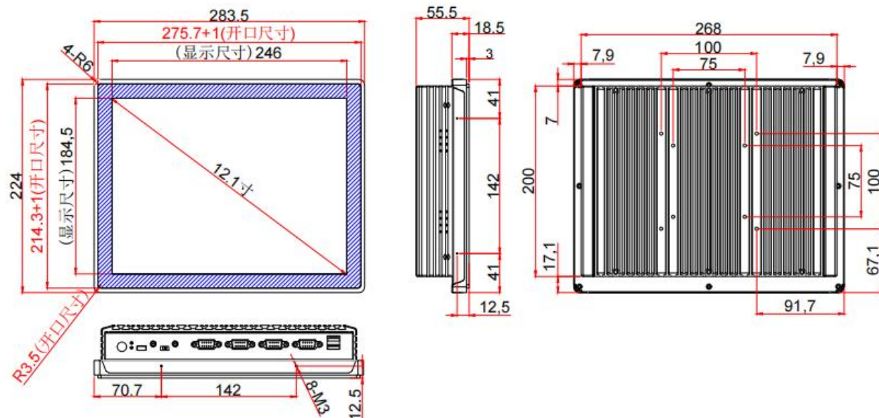
12.1寸内嵌式（散热款）-新
