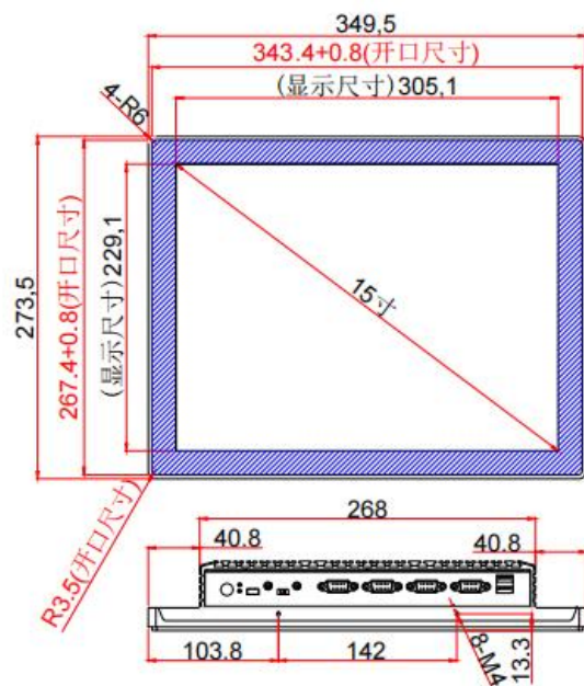
15寸内嵌式（全封闭）-新
