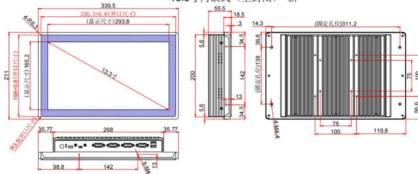
13.3寸内嵌式（散热款）-新
