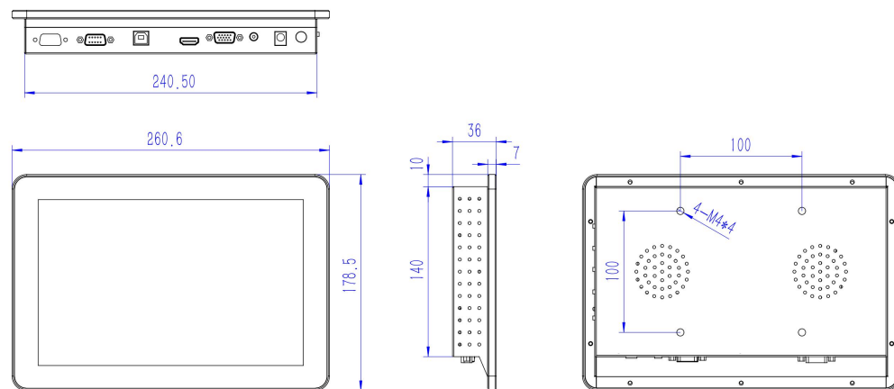
显示器图纸
